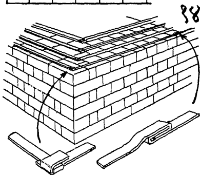
१२. Heading bond : बंदांची. १३. Herring bone bond : हेरिंग बोन. १४. Hoop-iron bond : हूप आयर्न.
